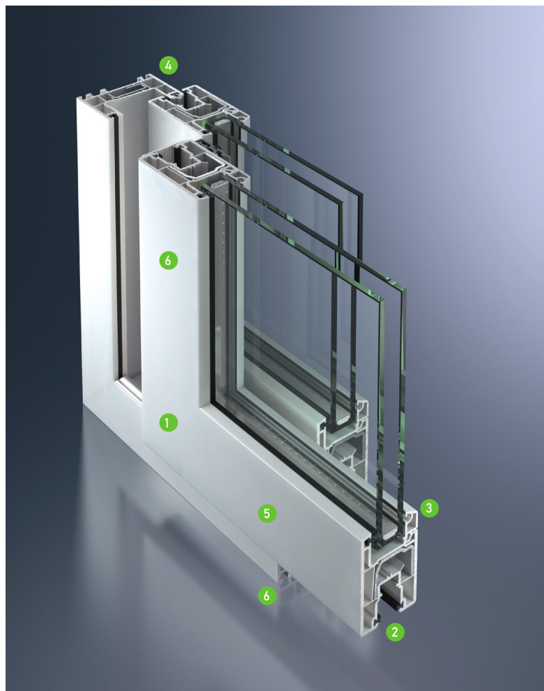
Sistema scorrevole in linea Schüco S 74
